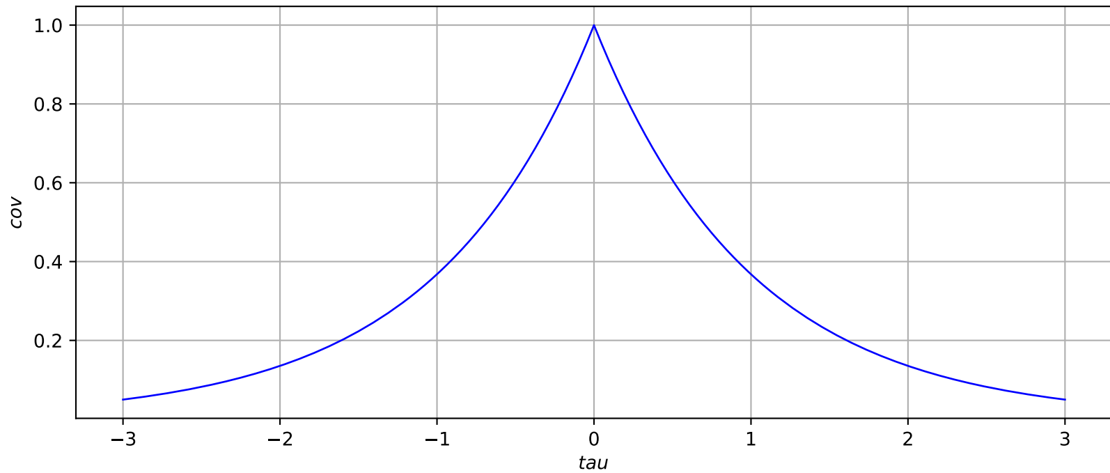
AbsoluteExponential(scale=[1], amplitude=[1])
